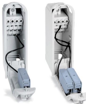
MORSETTIERA da PALO Pb Free – Feritoia 45x186
